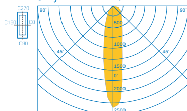
BeamTech s 1 svetelnou hlavou Úzký lúč v sklone 0°
