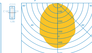
BeamTech 1 svetelná hlava Široký lúč v sklone 0°
